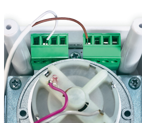
Фото 11. Подключение датчика к электроприводу
