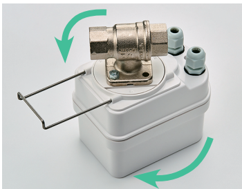
Фото 25. Крепление электропривода к шаровому крану с помощью металлической скобы
