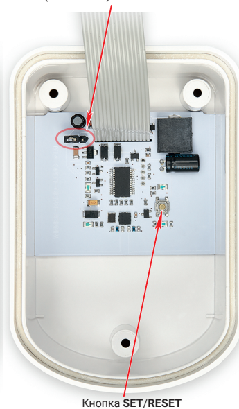
Фото 7. Элементы управления на внутренней стороне крышки шарового электропривода
