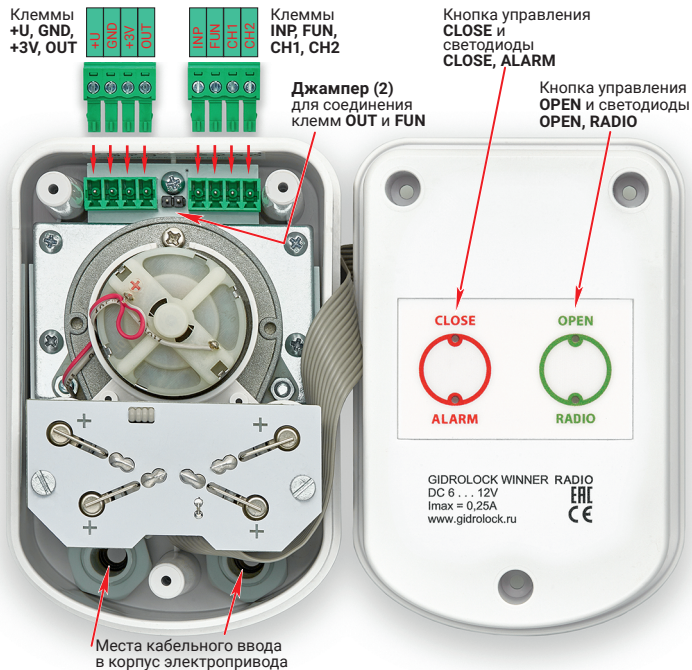
Фото 6. Электропривод управления шаровым краном со снятой крышкой
